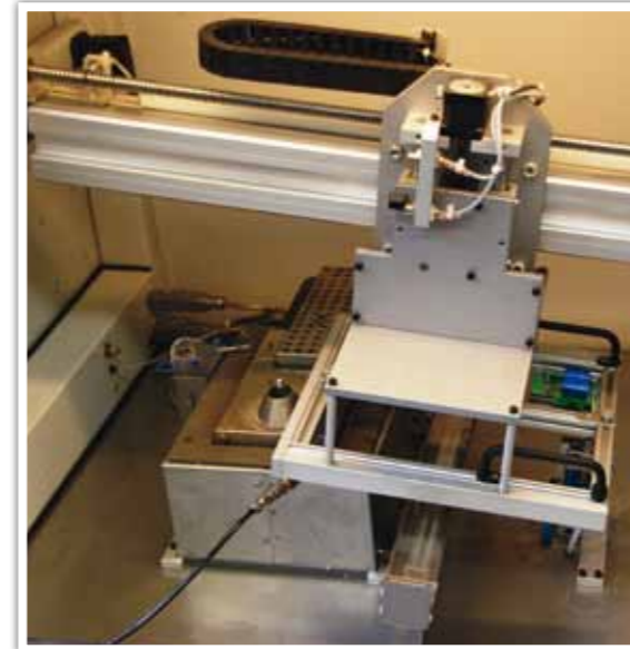
Zipa-Tec ECOSELECT 25 (selectieve soldeermachine)
