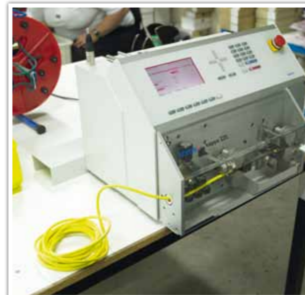
Kappa 220 kabelsnijmachine
